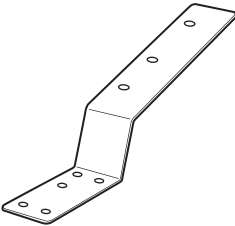
[9] フェンダーアッパー ブラケット LH/RH
